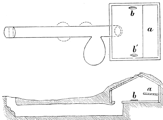
Fig. 43 a och b. Eskimåiskt vinterhus med gång, sedt i plan och genomskärning. Trakten af Point Barrow, nordvästra Nord-Amerika.
