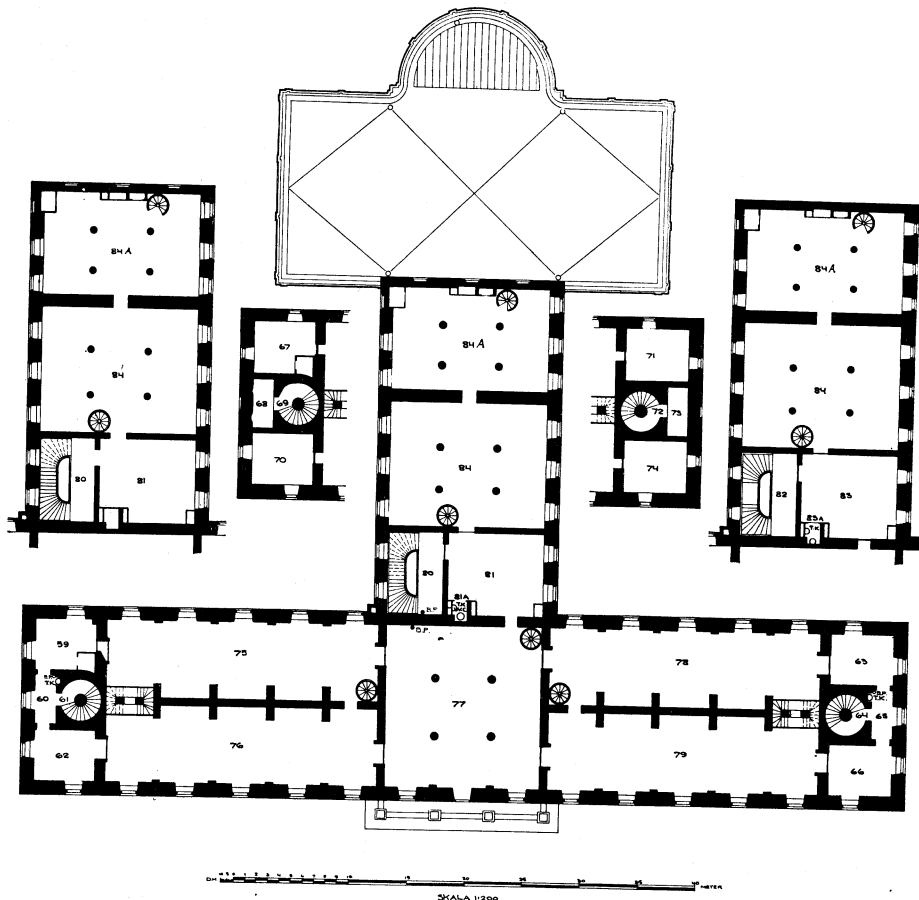
Fig. 5. Planer af våningen 1 tr. upp. — 59, 62—63, 66—67, 70—71, 74—79, 83, 84 och 84 A. Bokmagasin (59 och 67 med personhiss, 83 med bokhiss, 84 A med personhiss och bokhiss). 81. Amanuensrum och bokmagasin, med bokhiss. 60—61 och 64—65. Förstugor och trappor. (Dörrarna mellan 59—60, 60—62, 63—65, 65—66, 77—81 saknas på ritningen.) 80 och 82. Hufvudtrappan. (Ritningens dörröppningar mellan 80—81 och 81—84 i 1. galleriets plan existera icke.) 81 A och 83 A (gamla hisstrumman). Toalett och vattenposter.
